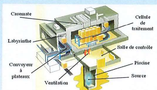
COUPE TYPE DE L'IRRADIATEUR INDUSTRIEL
